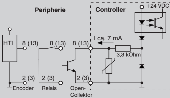
Eingangsschaltung Laser ON/OFF und Modeeingang
