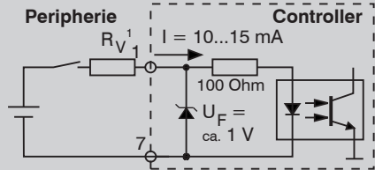
Schaltung Synchron Eingang
