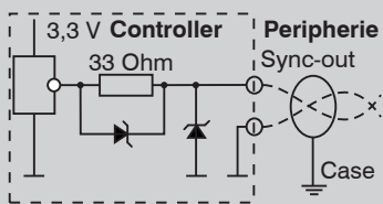
Schaltung Synchronausgang
