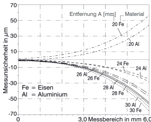
Abb. 5 Messunsicherheit in Abhängigkeit von Abstand A und Messobjektmaterial, DT3001-U6
