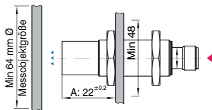
Abb. 4 Montage, Abmessungen in mm (nicht maßstabsgetreu)
