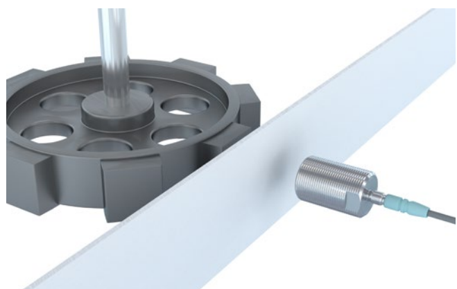
Vorgespannter Sensor zur Drehzahlmessung von Zahnrädern
