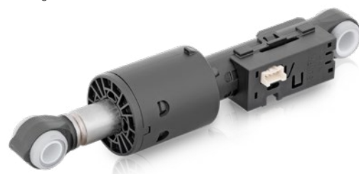
Anwendungsbeispiel: Integration in einen Waschmaschinendämpfer
