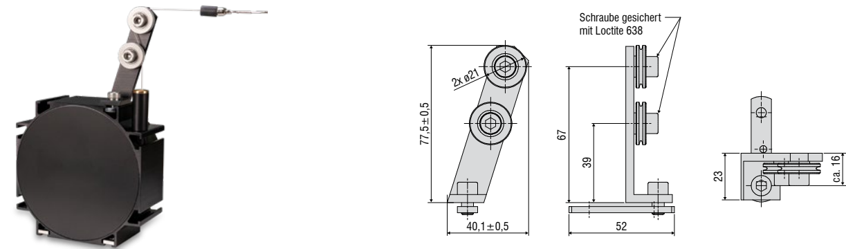
TR5-WDS(04) Integrierte Doppelumlenkrolle, 90° abgewinkelt, für Baureihe P115 mit Seildurchmesser 0,45 mm
