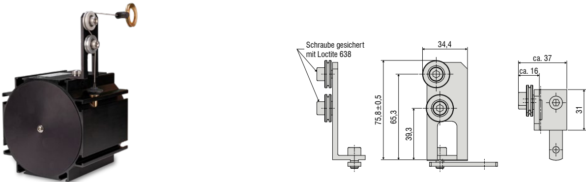
TR6-WDS(01) Integrierte Seilumlenkrolle für Baureihe P115 mit Seildurchmesser 1 mm
