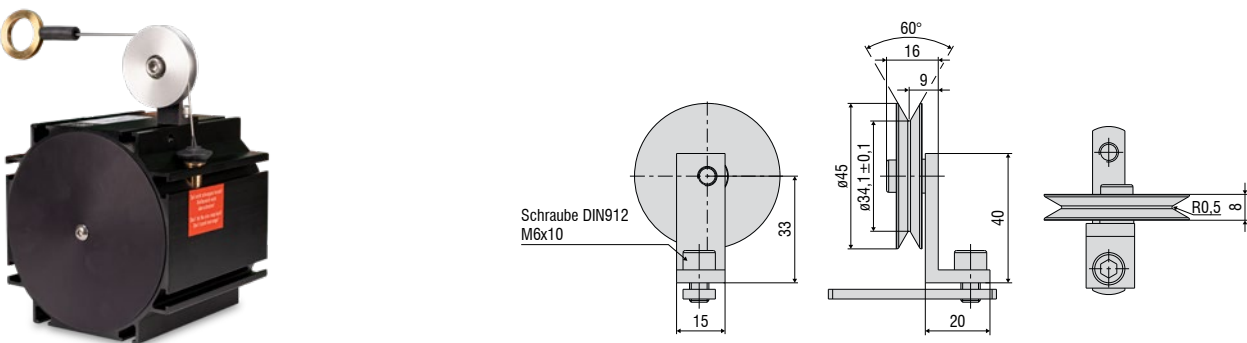
TR6-WDS(01) Integrierte Seilumlenkrolle für Baureihe P115 mit Seildurchmesser 1 mm
