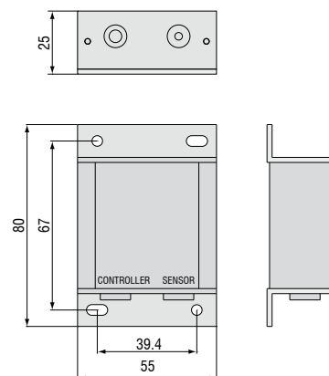
CP6001 kapazitiver Vorverstärker
