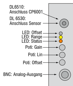
DL6530/6510 Frontansicht
