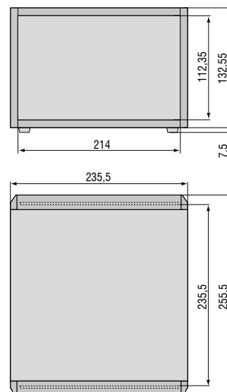
Controller DT6530C 2-Kanal-Ausführung
