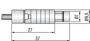
Stecker Typ B
