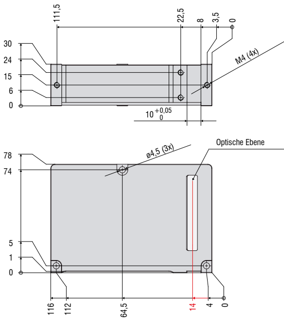
Empfänger
