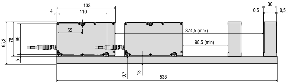
Lichtquelle und Empfänger mit Montageschiene
