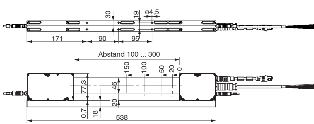
Abb. 2 Maßzeichnung Lichtquelle und Empfänger mit Montageschiene, Abmessungen in mm, nicht maßstabsgetreu
