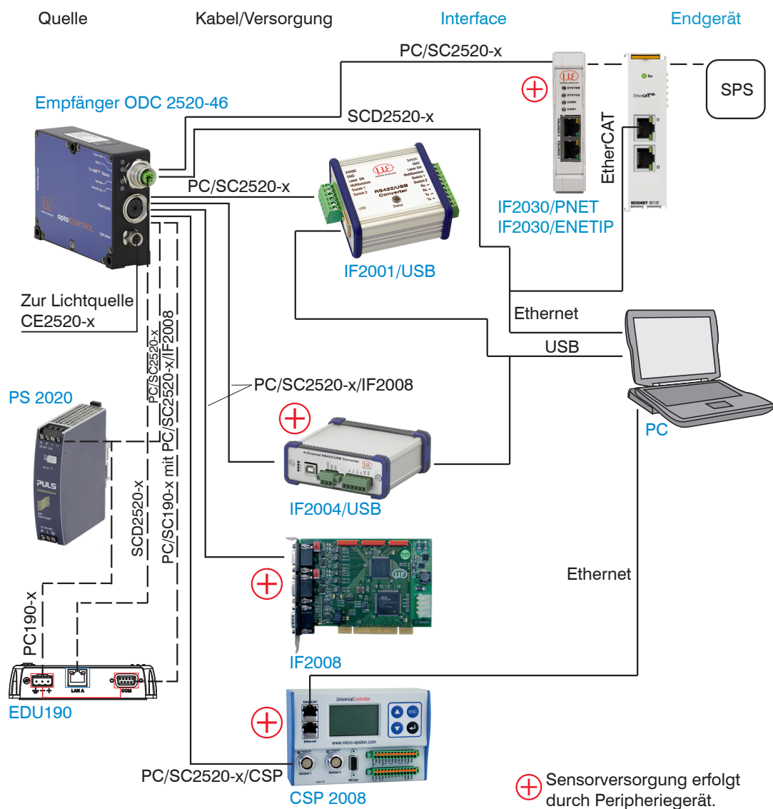
Abb. 7 Anschlussbeispiele am optoCONTROL 2520-46
