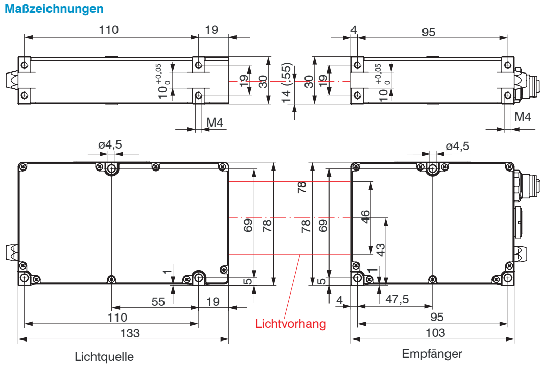
Abb. 1 Maßzeichnung Lichtquelle und Empfänger, Abmessungen in mm, nicht maßstabsgetreu
