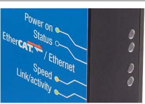
Abb. 6 LEDs an der Ethernet/ EtherCAT-Buchse
