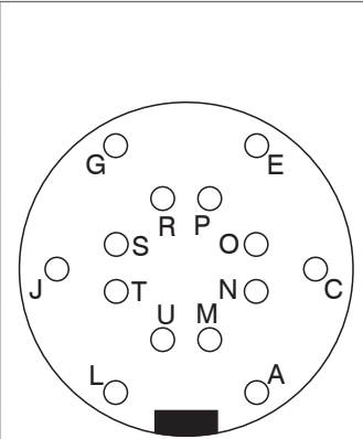
14-pol. Kabelstecker Ansicht Lötseite
